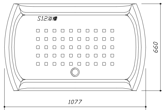
< 浴槽詳細図 >
