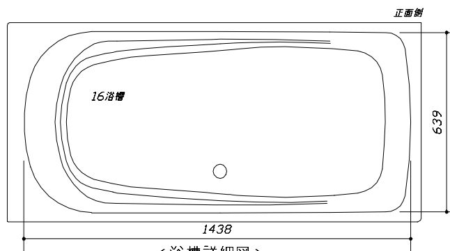
<浴槽詳細図>
