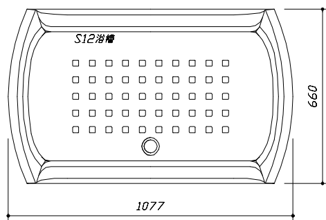
<浴槽詳細図>
