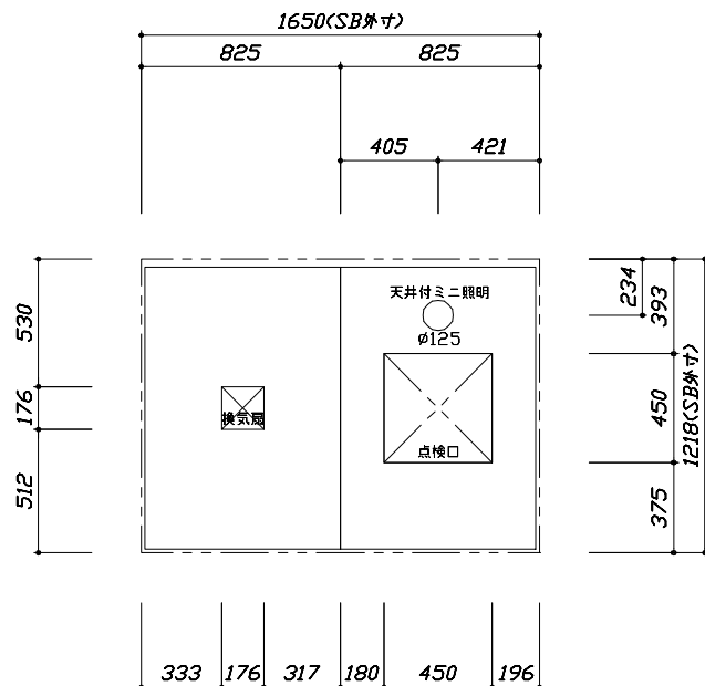
<天井伏図>
