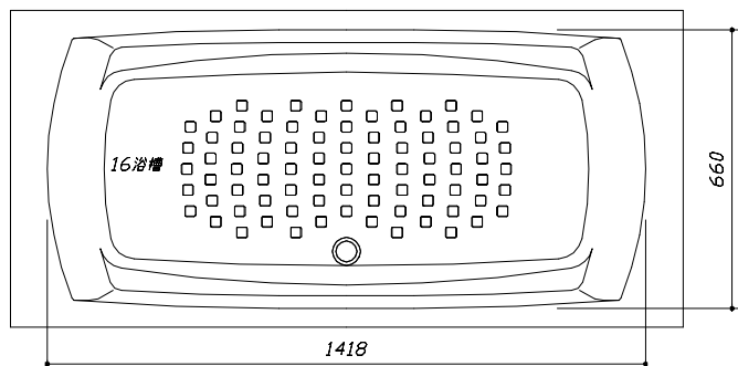
<浴槽詳細図>
