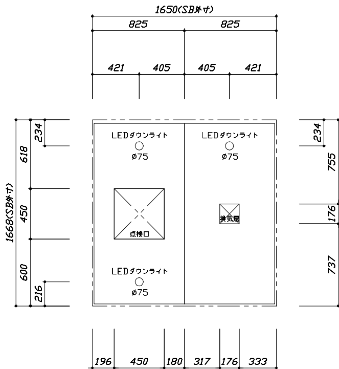
<天井伏図>
