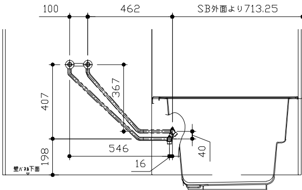
＜給水給湯管取合詳細図＞
