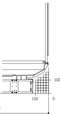
A矢視
