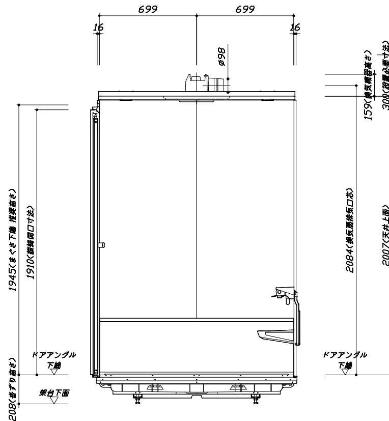
< 浴槽側面図 >
