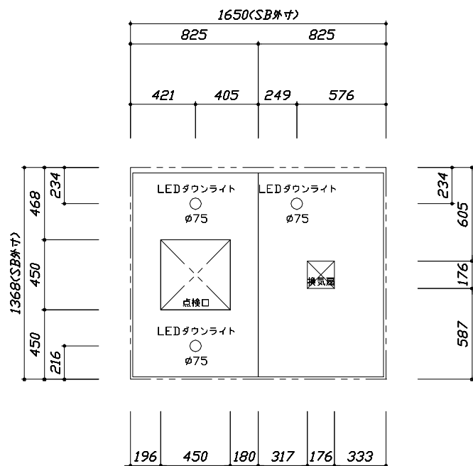
<天井伏図>
