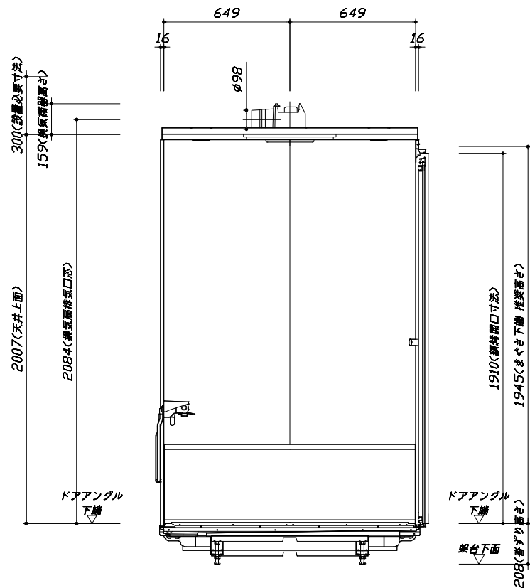
< 浴槽側面図 >
