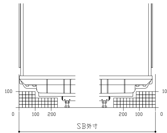
F矢視
