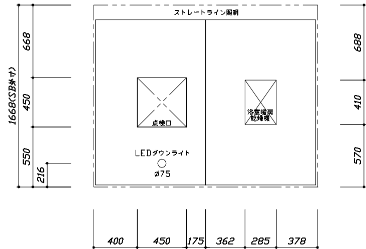
<天井伏図>
