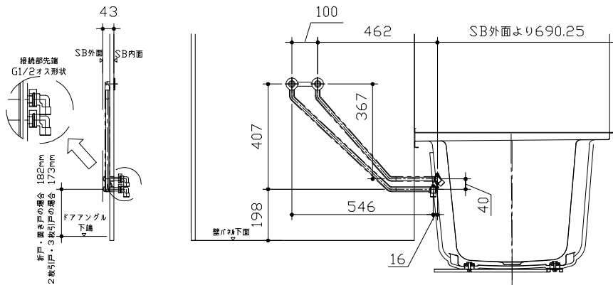
〈給水給湯管取合詳細図〉
