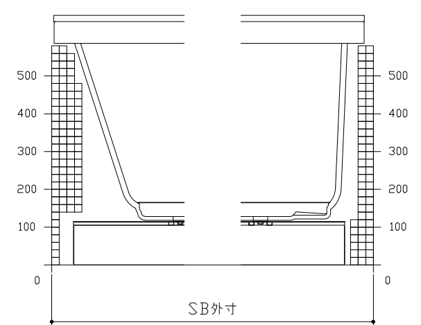
F矢視
