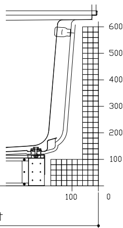
A矢視
