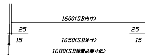
<平面図>
