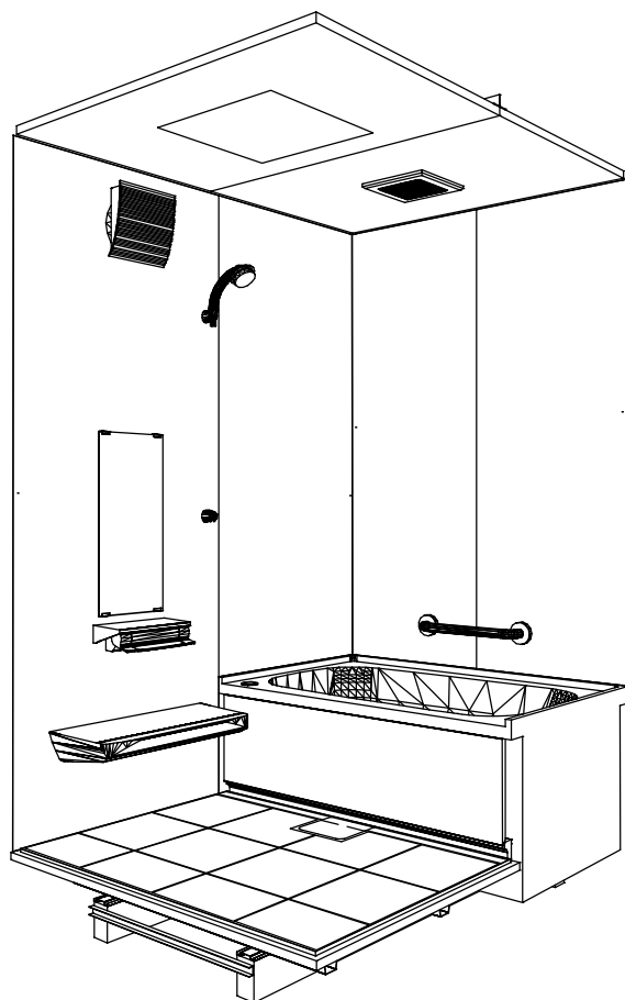
パース
