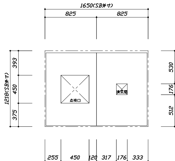
<天井伏図>
