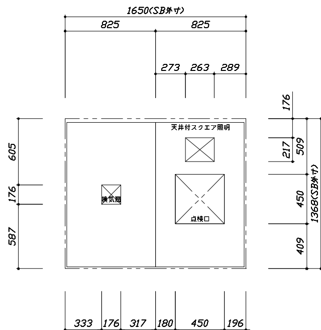
< 天井伏図 >
