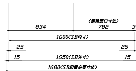
< 平面図 >
