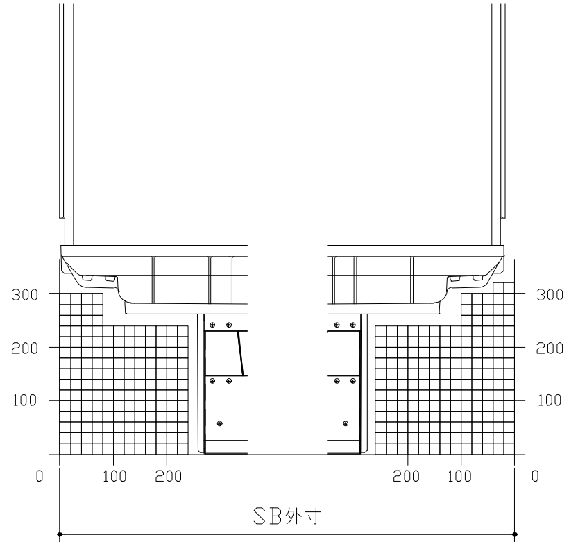
F矢視
