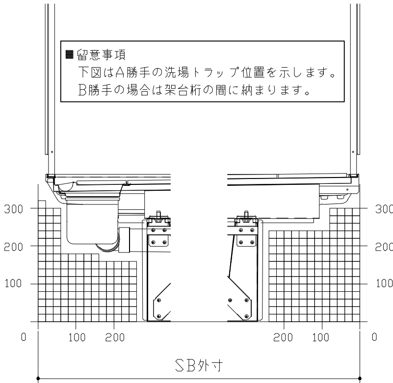
D矢視
