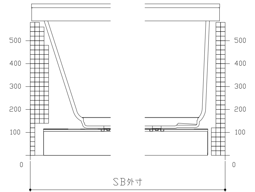
F矢視
