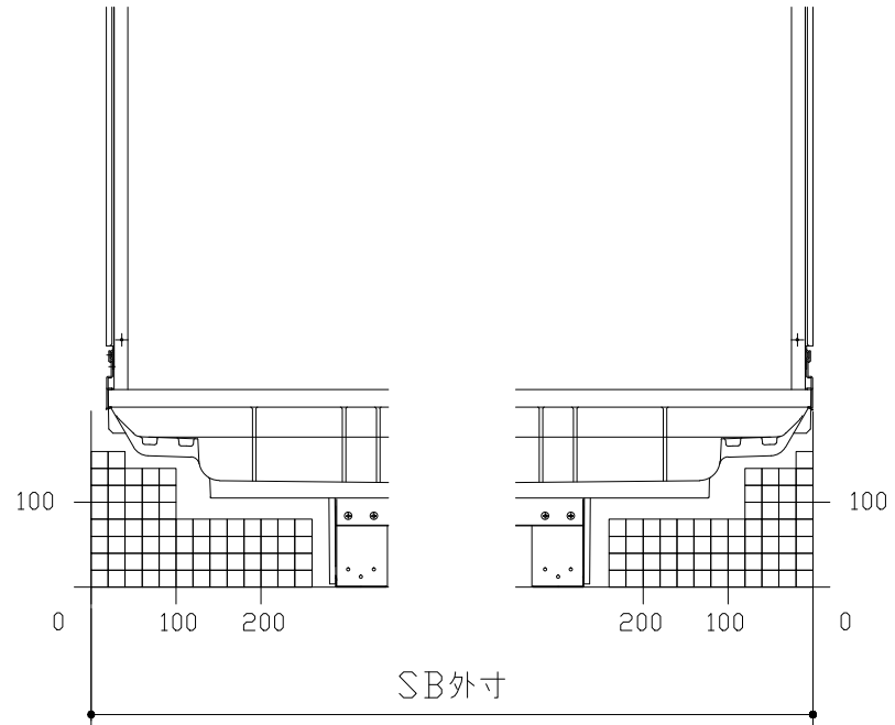
E矢視
