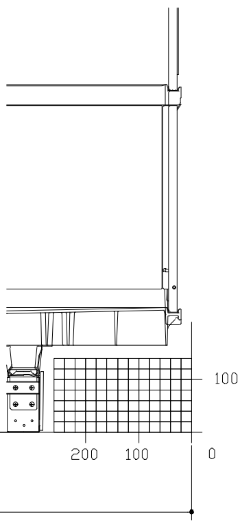
D矢視
