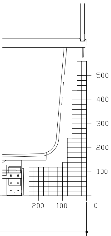
F矢視
