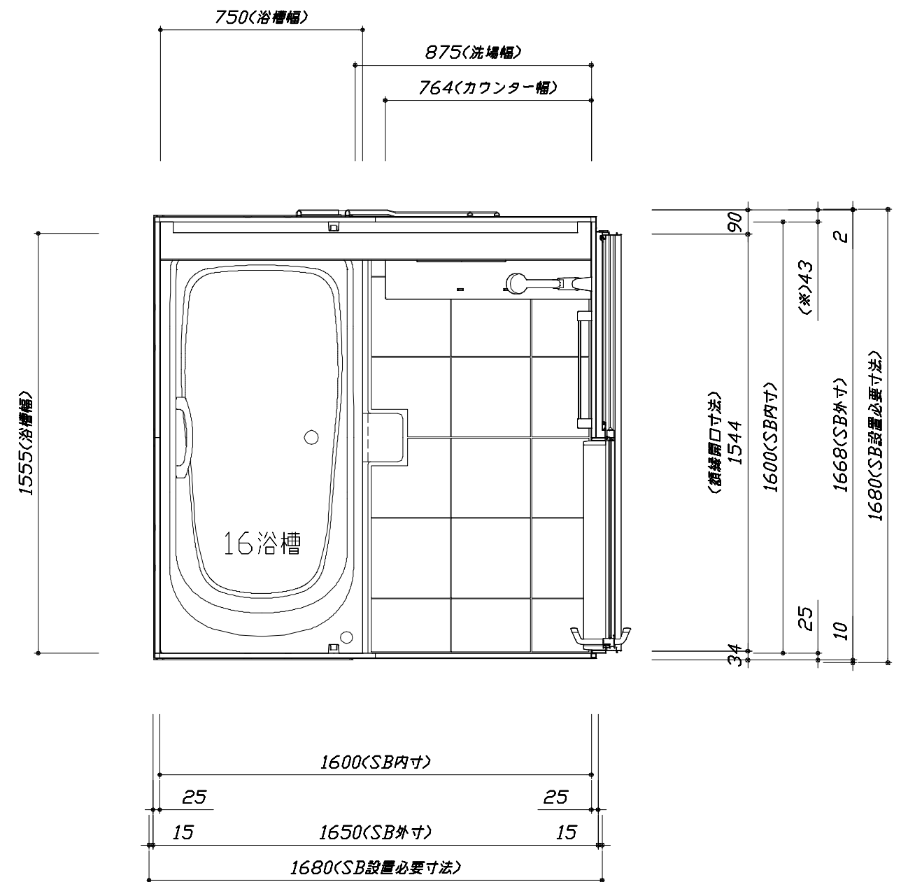
< 平面図 >
