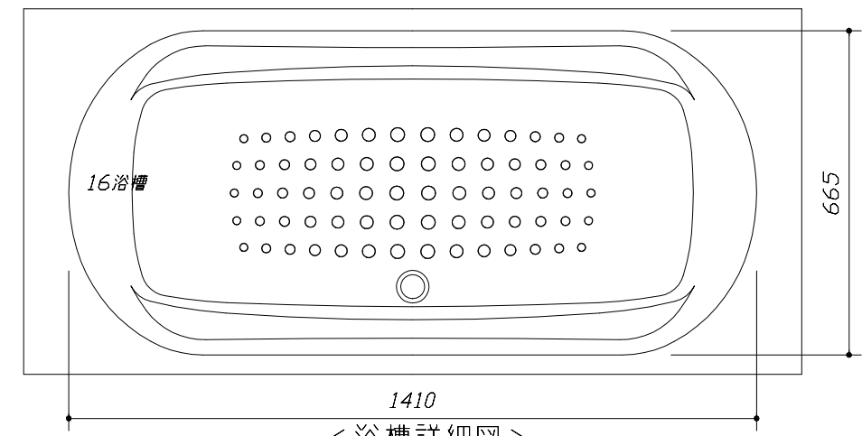
< 浴槽詳細図 >
