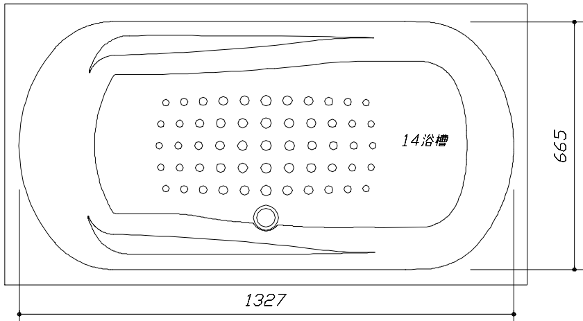
< 浴槽詳細図 >
