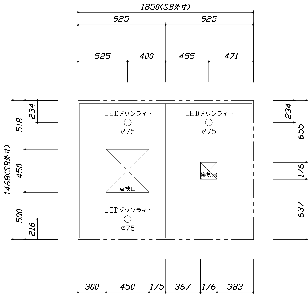
< 天井伏図 >
