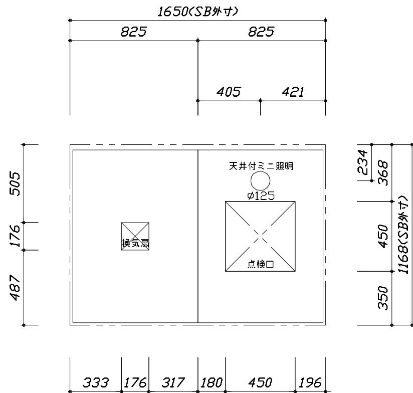
< 天井伏図 >
