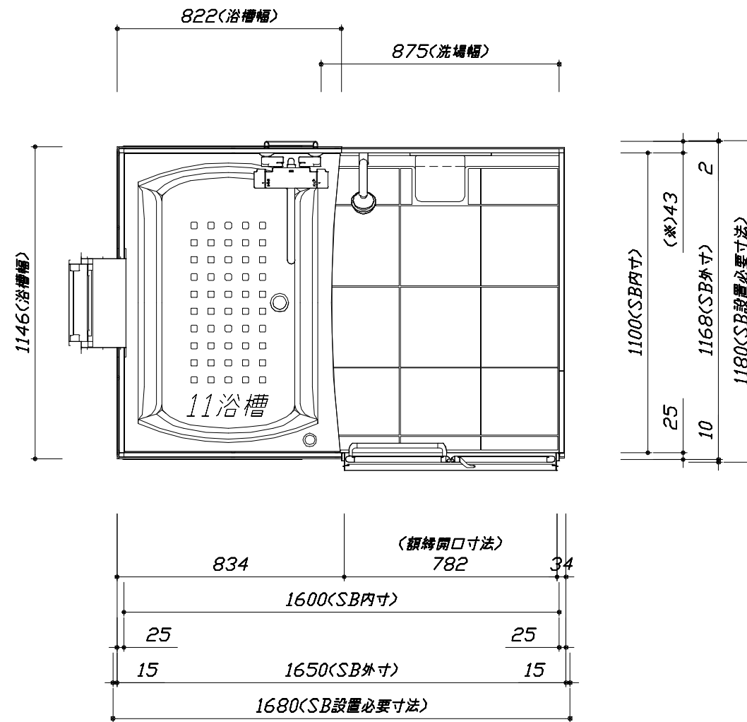
< 平面図 >
