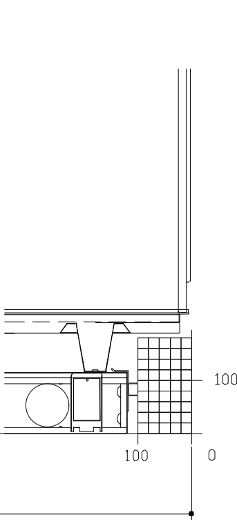
B矢視
