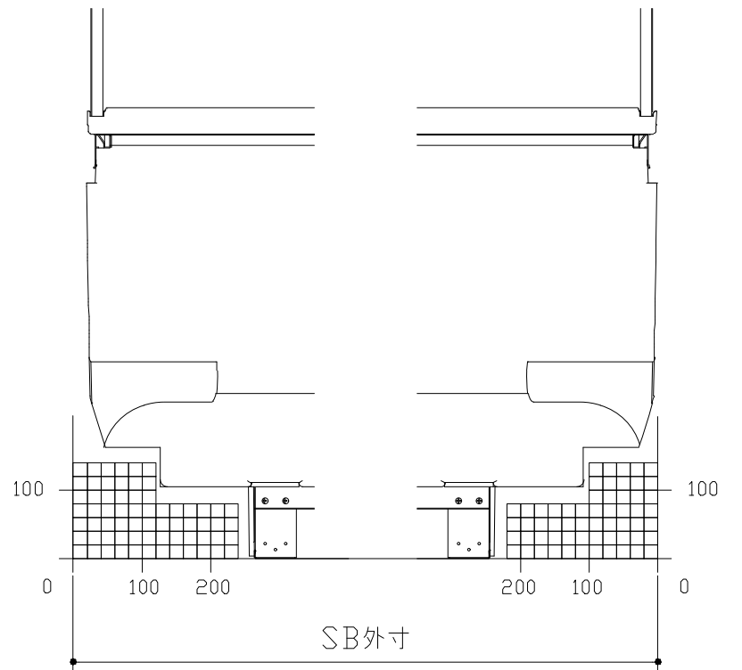
E矢視
