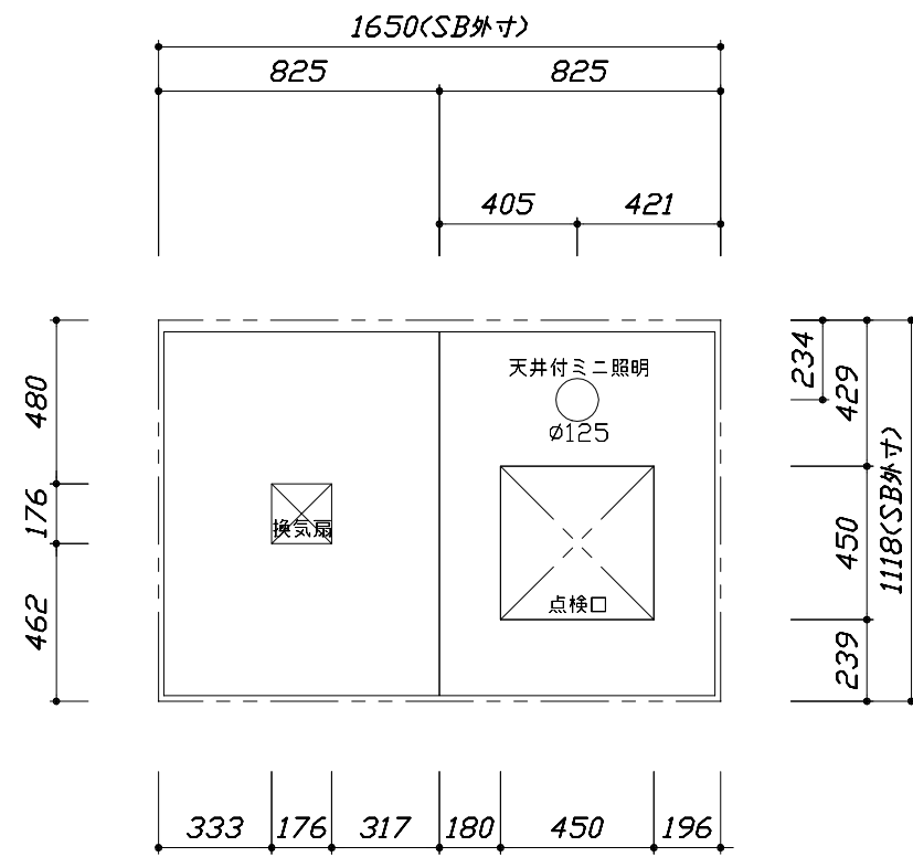
< 天井伏図 >
