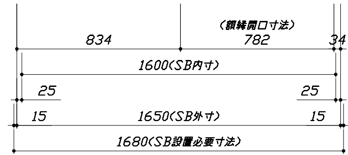
< 平面図 >
