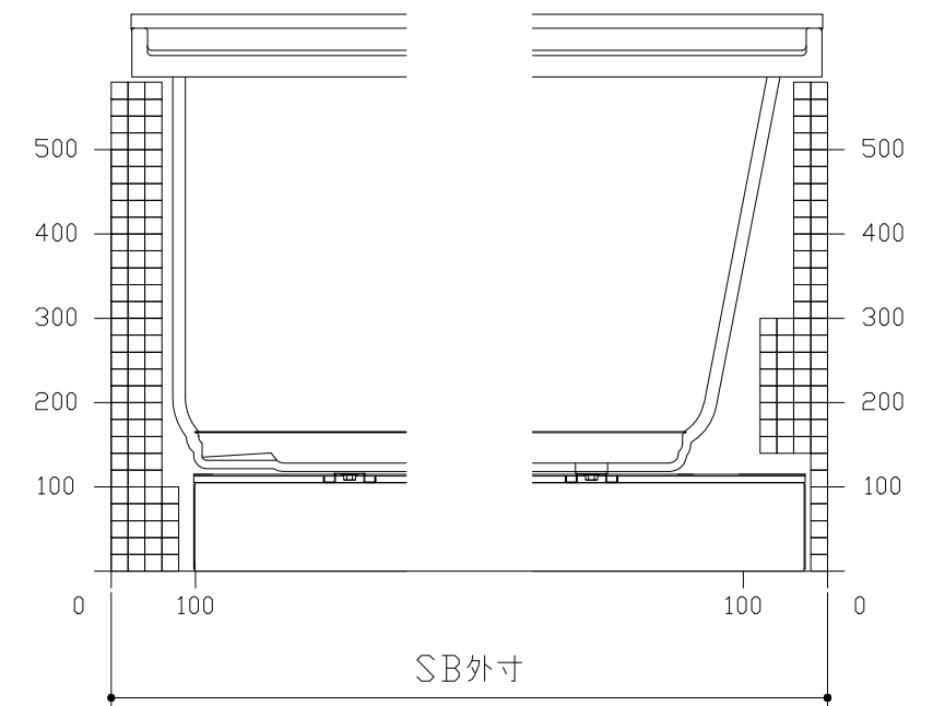
C矢視
