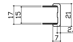
断面図
