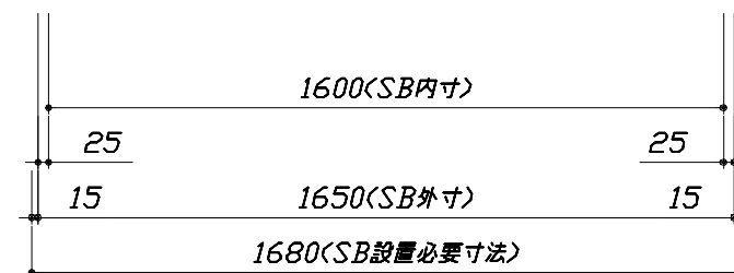
< 平面図 >
