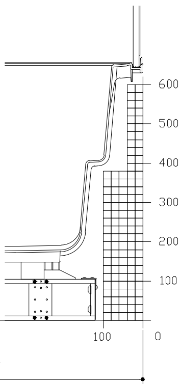
A矢視
