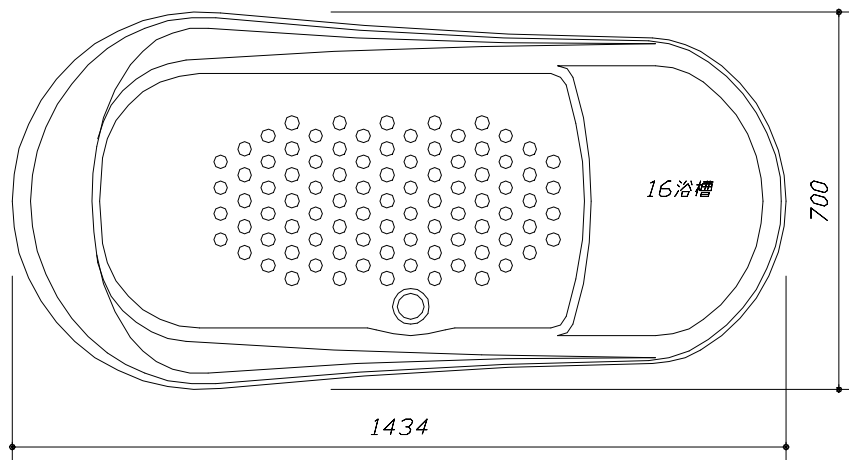
< 浴槽詳細図 >
