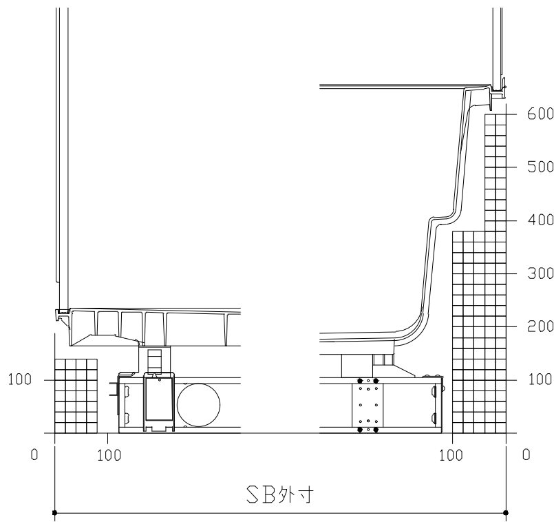
B矢視
