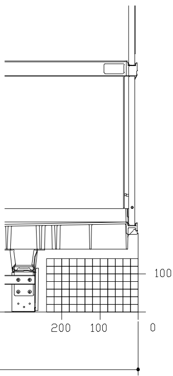
C矢視
