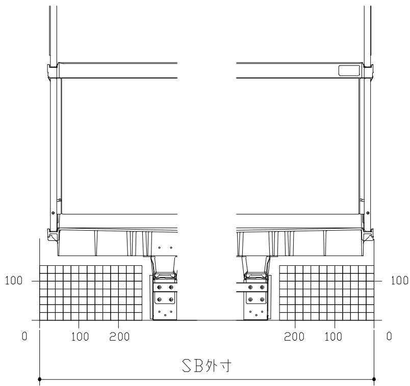
D矢視
