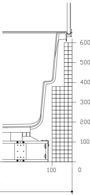
A矢視
