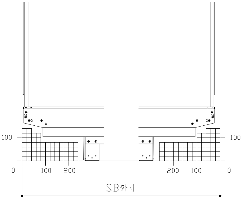
F矢視
