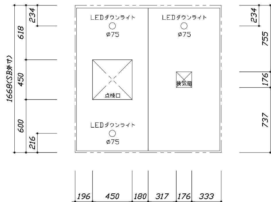
<天井伏図>
