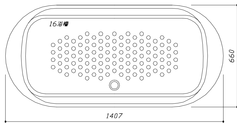
< 浴槽詳細図 >
