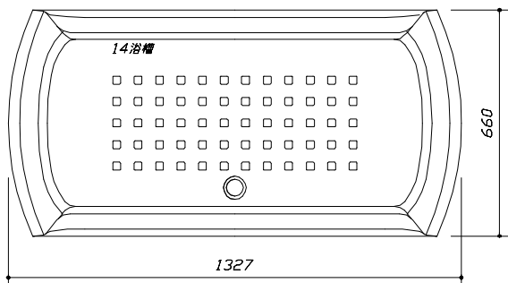
<浴槽詳細図>
