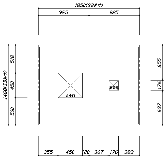
<天井伏図>
