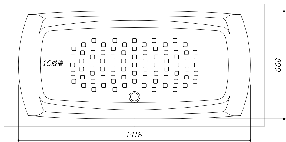
<浴槽詳細図>
