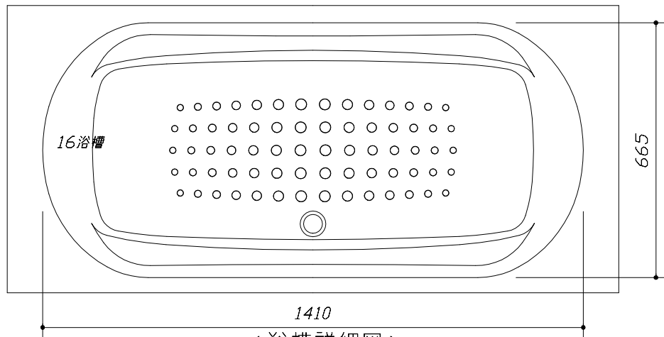
< 浴槽詳細図 >
