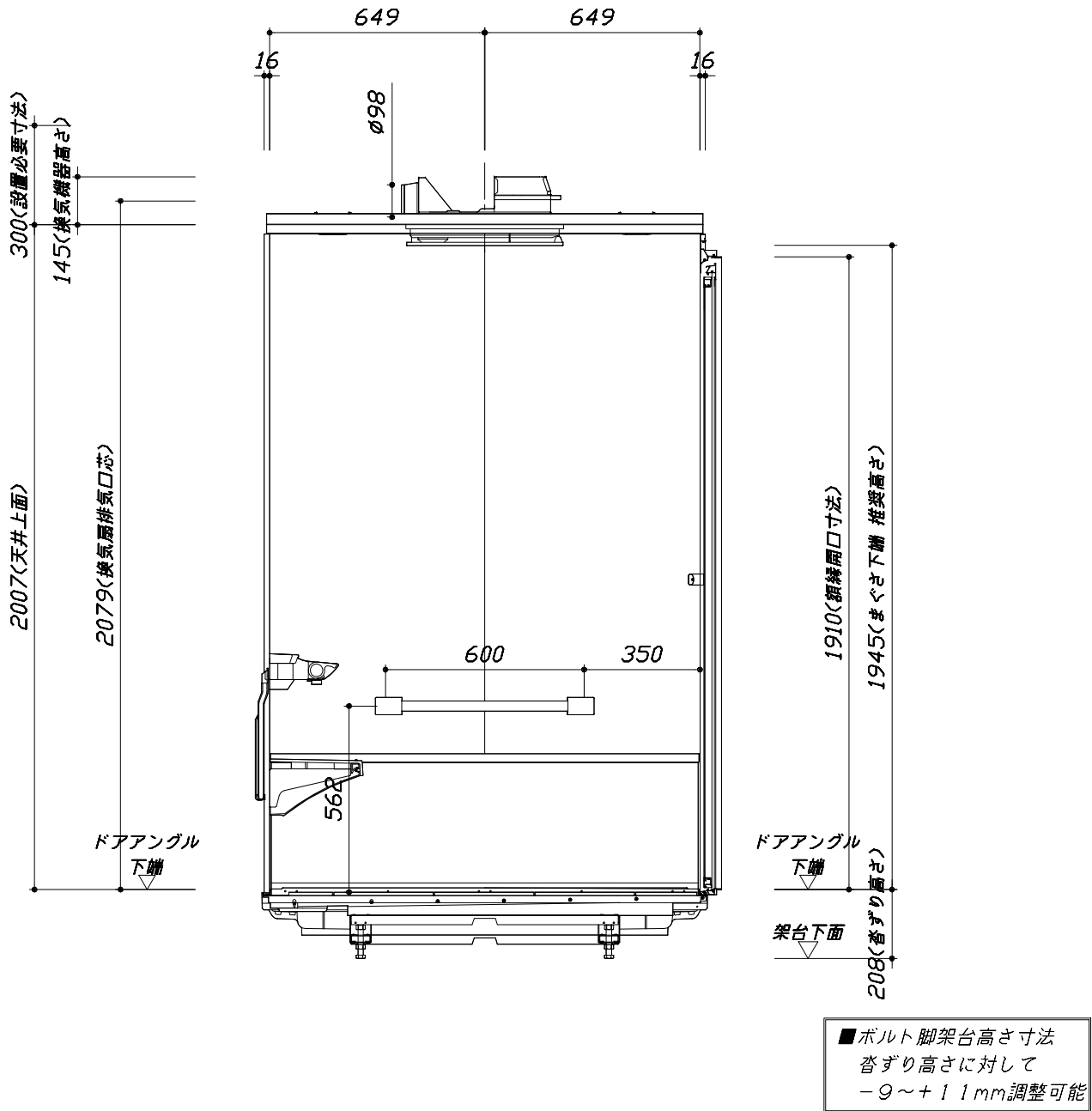
< 浴槽側面図 >
