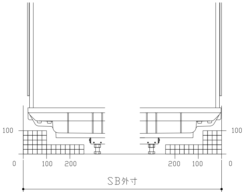
E矢視
