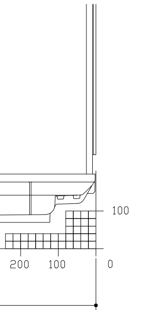
F矢視
