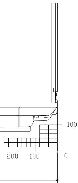
F矢視
