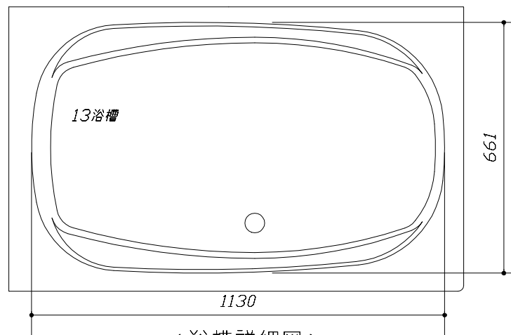
< 浴槽詳細図 >
