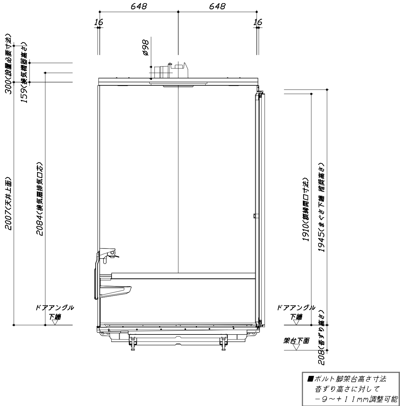
< 浴槽側面図 >
