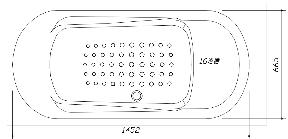
<浴槽詳細図>
