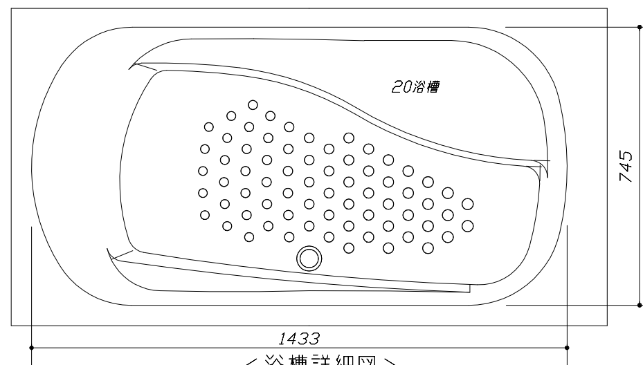
< 浴槽詳細図 >
