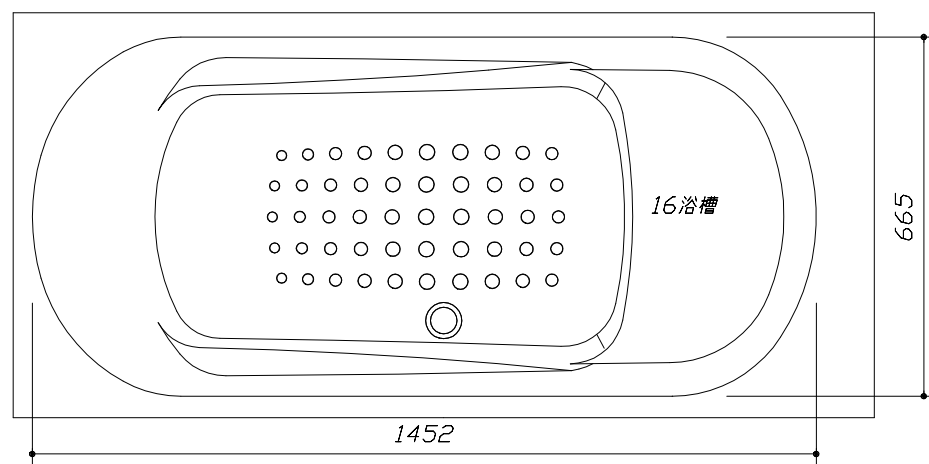
<浴槽詳細図>
