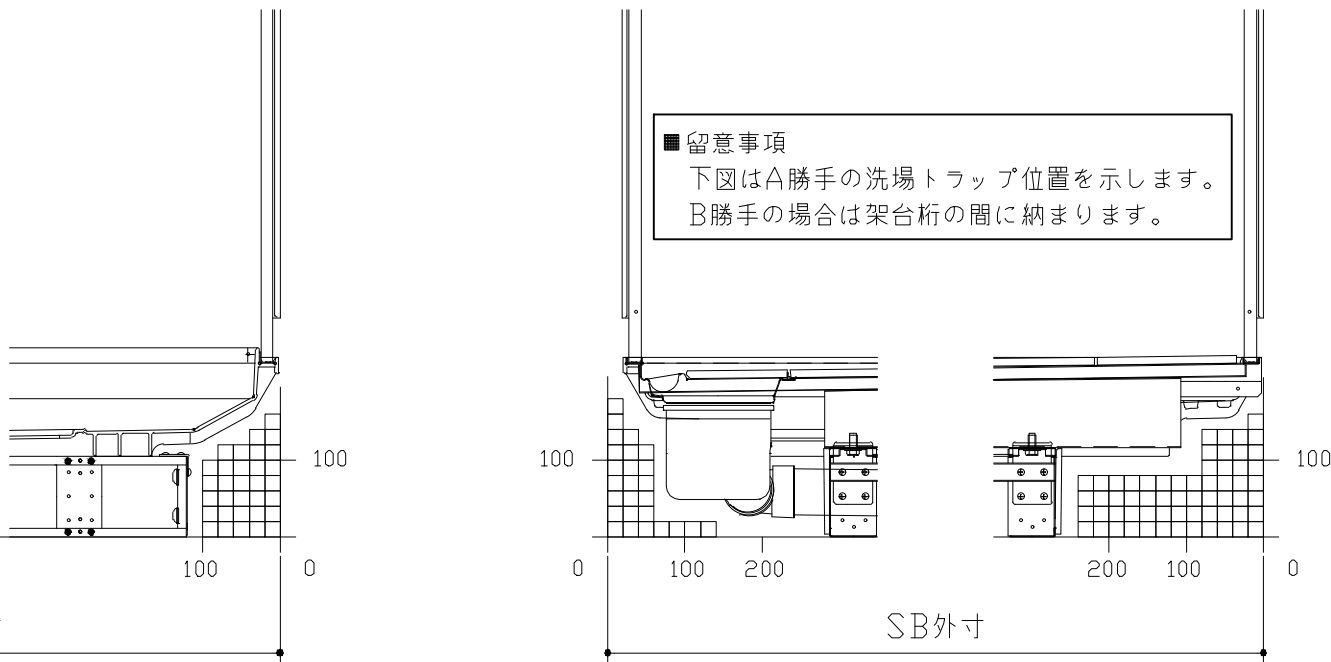
D矢視
