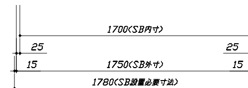
< 平面図 >
