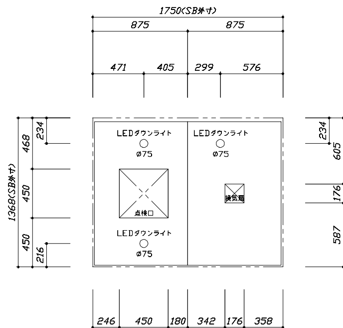
< 天井伏図 >
