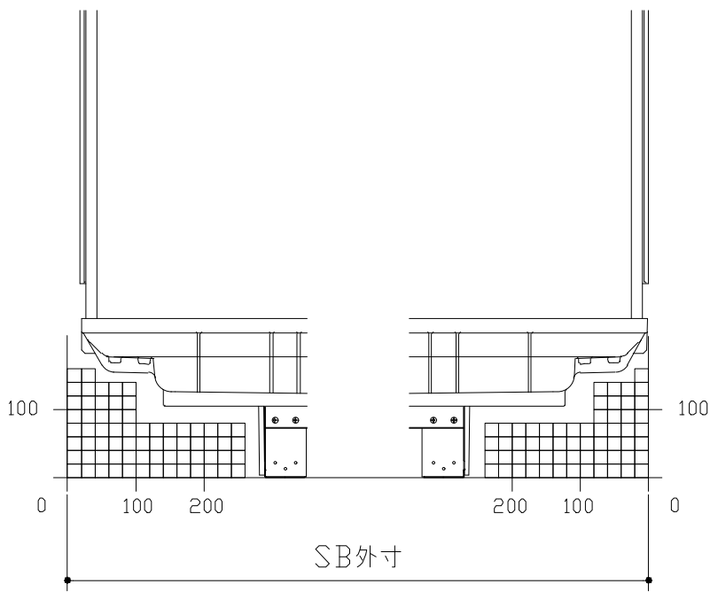
D矢視
