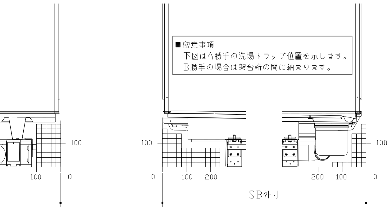
B矢視
