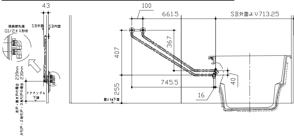
〈給水給湯管取合詳細図〉
