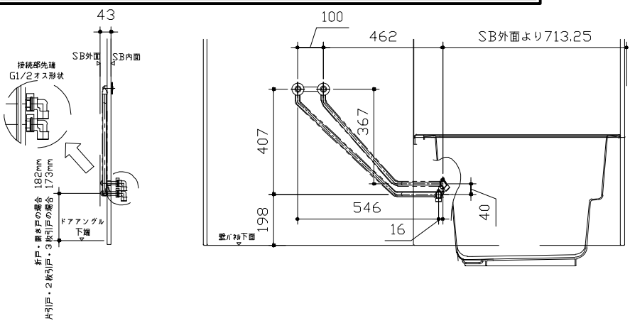
〈給水給湯管取合詳細図〉
