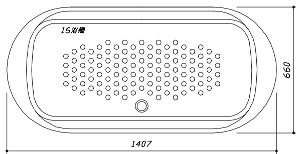
< 浴槽詳細図 >
