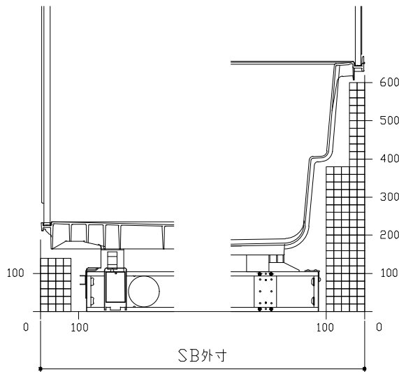
B矢視
