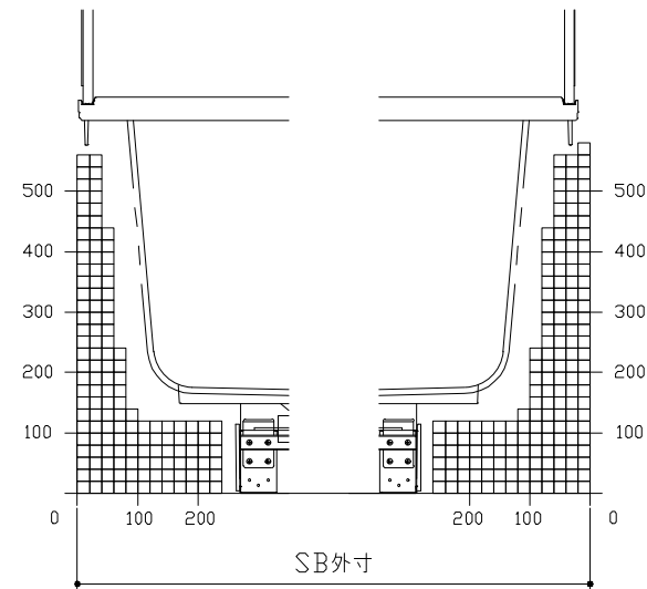
F矢視
