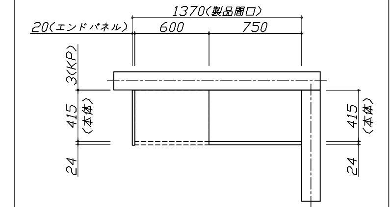
上台伏せ図
