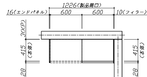
上台伏せ図
