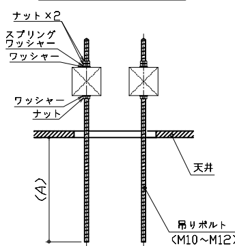
吊ボルト 取付参考図
