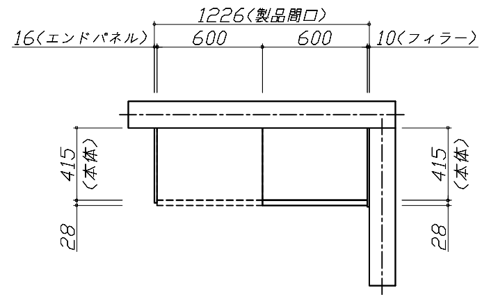
上台伏せ図
