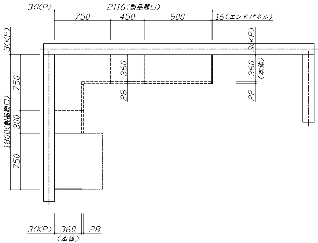
上台伏せ図
