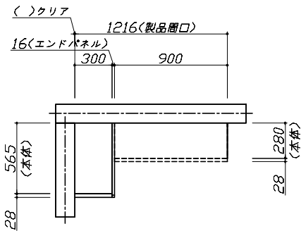
上台伏せ図
