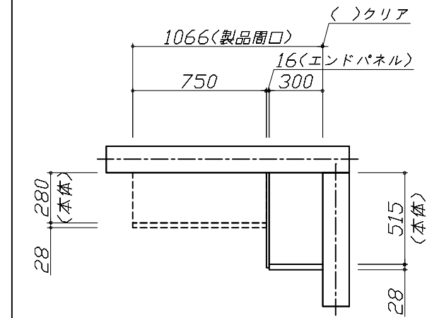
上台伏せ図
