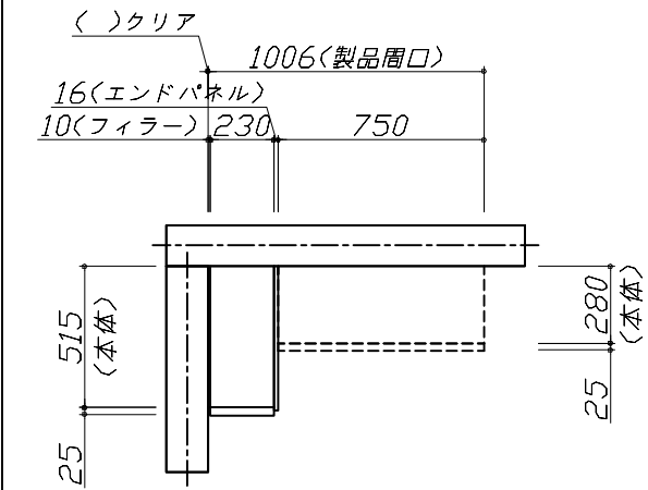
上台伏せ図
