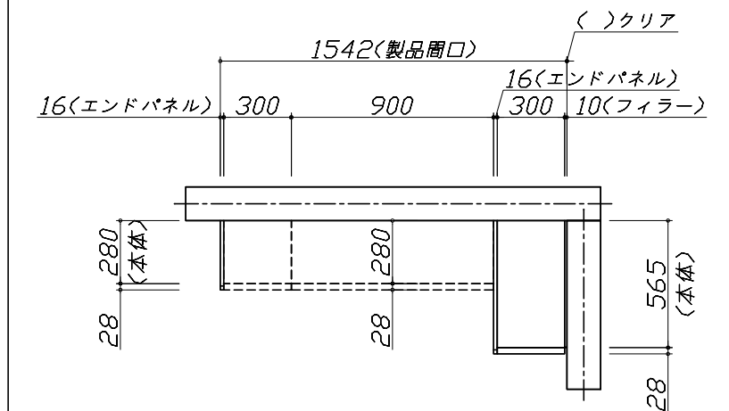
上台伏せ図
