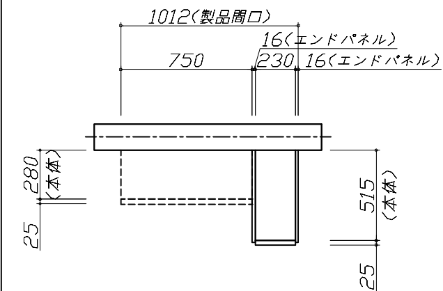
上台伏せ図
